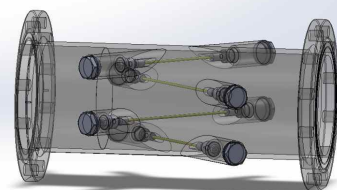
DN200~DN300 4-path
