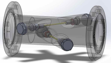
DN50~DN100 2-path
